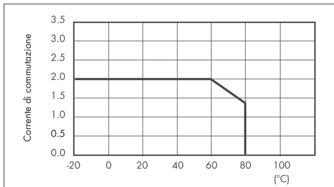
L 34 - Corrente di commutazione in funzione della temperatura ambiente SSR con uscita 2A (DC e AC)
