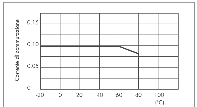
L 34 - Corrente di commutazione in funzione della temperatura ambiente SSR con uscita 0.1A (DC)
