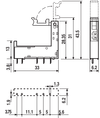
Vista lato rame
