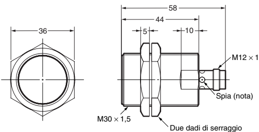
E2A-M30KS15-M1-□□/E2A-S30KS15-M1-□
