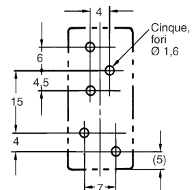
Disposizione terminali (vista dal basso)
