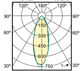
(cd/1000lm) 0° — 0-180° — 90-270°
