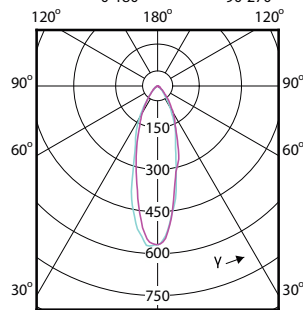
(cd) 0° — 0-180° — 90-270°
