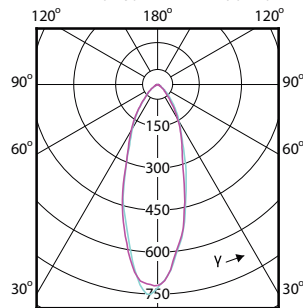
(cd) 0° — 0-180° — 90-270°
