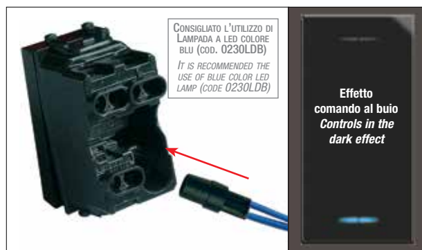
Inserimento lampadina di segnalazione Lamp insertion
