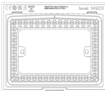
Vista posteriore
