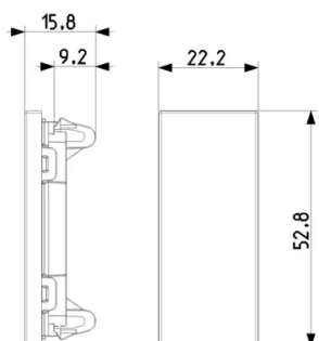
Vista ingombri
