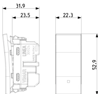
Vista ingombri
