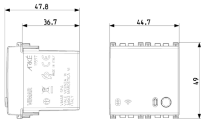
Vista ingombri
