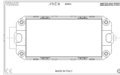
Vista posteriore
