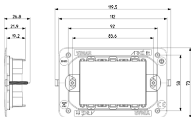
Vista ingombri
