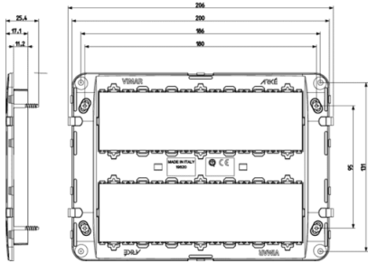
Vista ingombri
